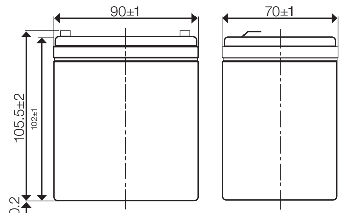
Faston tab : 250
