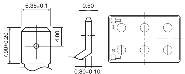
Faston tab : 250
