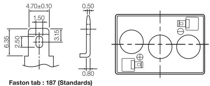
Faston tab : 187 (Standards)
