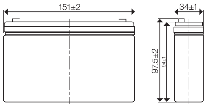
Faston tab : 187 (Standards)
